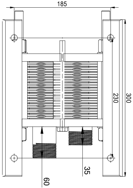
Quota di serraggio (Q)mm - Numero Piastre x (2.35 + sp. piastre)
