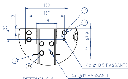
DETTAGLIO A
