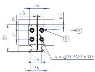
SEZIONE D-D
