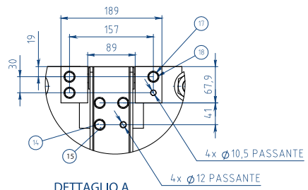
DETTAGLIO A
